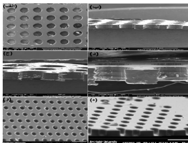
شکل ۲: تصاویر SEM به دست آمده از میکرو فیلترهای PDMS، (الف) و (ب) نمای سطح بالا و سطح مقطع جانبی میکرو فیلتر ۵۰۰، (ج) و (د) نمای سطح بالا و سطح مقطع جانبی میکرو فیلتر ۳۰۰، (و) و (ه) نمای سطح بالا و سطح مقطع جانبی میکرو فیلتر ۱۰
