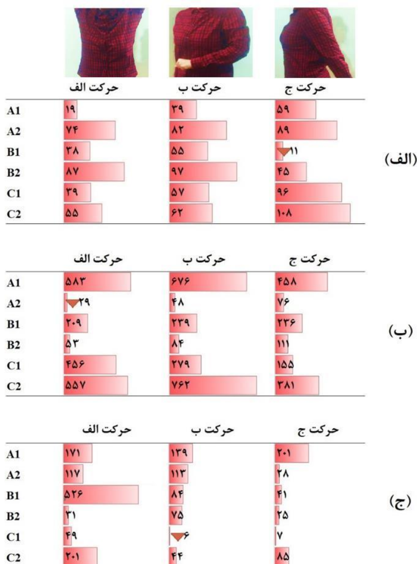
شکل ۳: مقادیر شیب نمودار ولتاژ-زمان ( \times 10000 ) در حین انجام حرکات مختلف: (الف) نخ فلزی در پایین کاپ، (ب) نخ فلزی در پایین نواری پشتی، (ج) نخ فلزی در پایین سه‌گوش میانی
