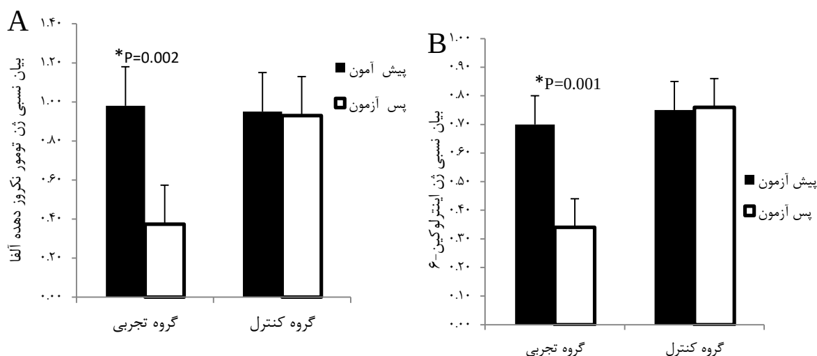
شکل ۴: میزان بیان ژن IL-6 (A) و TNF-α (B) در PBMC گروه‌های کنترل و تجربی با استفاده از روش Real Time-PCR پیش و پس از ۱۲ هفته مداخله. داده‌ها به صورت میانگین \pm انحراف معیار ارائه شده است. برای مقایسه گروه‌ها از آنالیز واریانس با اندازه‌گیری‌های مکرر استفاده شد. سطح معنی‌داری پذیرفته شده P<0/05 در نظر گرفته شد.
