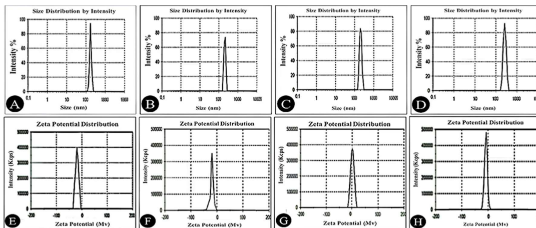
شکل ۴: اندازه و پتانسیل نانوذرات (A تا D) اندازه نانوکپسول‌های PCPF، PCPF/siRNA، PCPF/PTX و PCPF/siRNA/PTX؛ پتانسیل زتای نانوکپسول‌های PCPF، PCPF/siRNA، PCPF/PTX و PCPF/siRNA/PTX Nps؛ (E تا H) Zeta potential of PCPF، PCPF/siRNA، PCPF/PTX، and PCPF/siRNA/PTX NPs.
