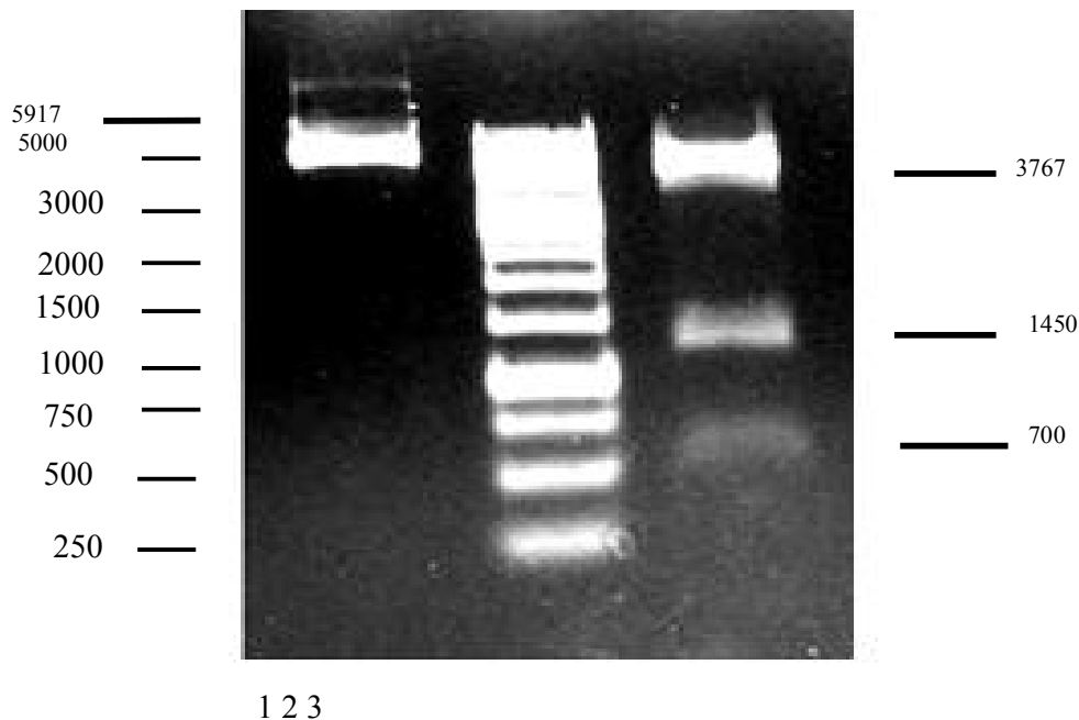
شکل ۵: محصول هضم محدودالایر قطعه F(ab')_2 -PET32-EK/LIC توسط آنزیم‌های NCOI و XbaI که سه قطعه را ایجاد می‌کند.
