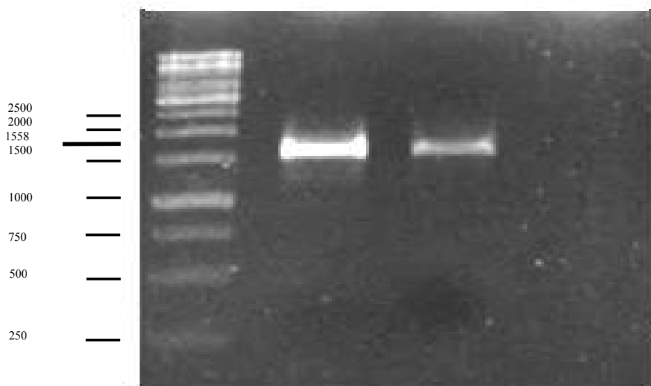
شکل ۳: محصولات مربوط به کلونی PCR، با استفاده از پرایمرهای اختصاصی حامل PET-32 EK/LIC.
